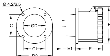
Ölçüler (mm)
