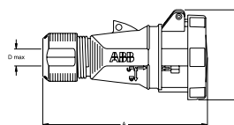
Ölçüler (mm)
