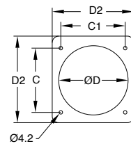
Ölçüler (mm)
