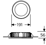
Tavan Kesim Ölçüsü: Ø 153
