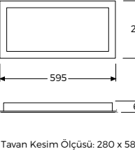
Tavan Kesim Ölçüsü: 280 x 580
