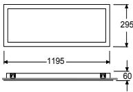
Tavan Kesim Ölçüsü: 280 x 1180
