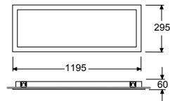
Tavan Kesim Ölçüsü: 280 x 1180
