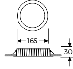
Tavan Kesim Ölçüsü: Ø 140
