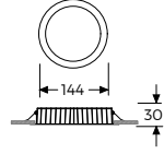
Tavan Kesim Ölçüsü: Ø 120
