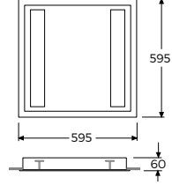
Tavan Kesim Ölçüsü: 580 x 580
