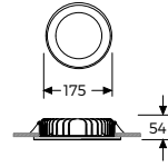
Tavan Kesim Ölçüsü: Ø 141
