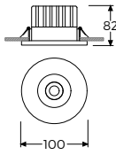
Tavan Kesim Ölçüsü: Ø72
