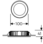
Tavan Kesim Ölçüsü: Ø 67
