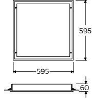
Tavan Kesim Ölçüsü: 580 x 580
