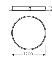
Tavan Kesim Ölçüsü: Ø 1192
