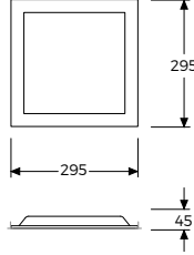
Tavan Kesim Ölçüsü: 280 x 280
