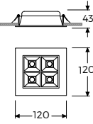
Tavan Kesim Ölçüsü: 110 x 110
